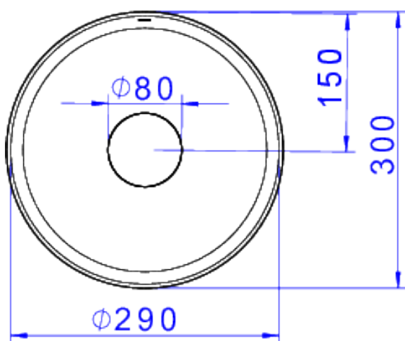
Desenho Técnico
