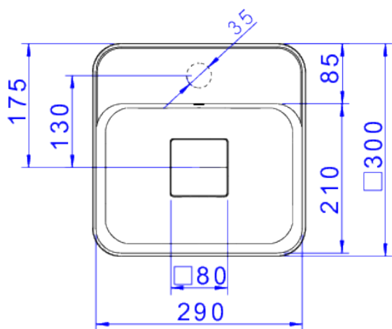
Desenho Técnico
