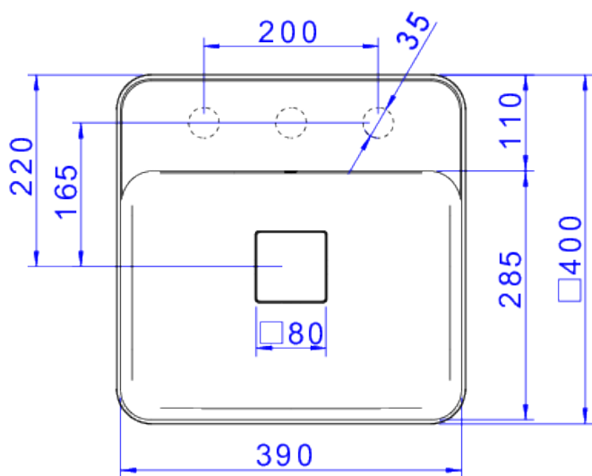
Desenho Técnico
