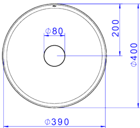
Desenho Técnico
