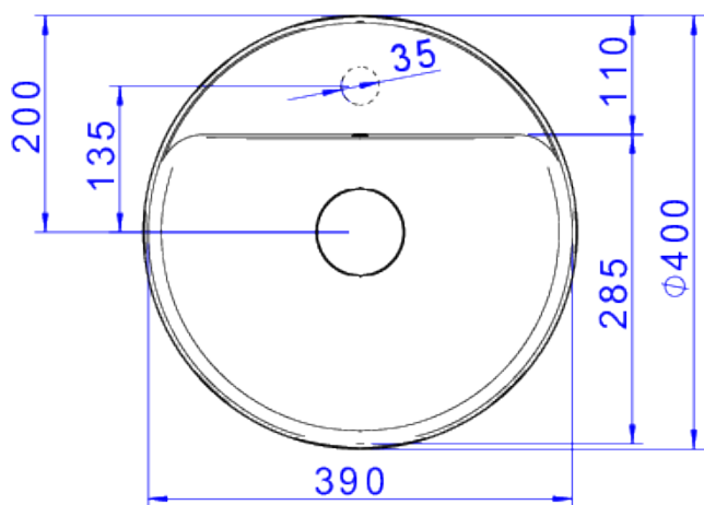
Desenho Técnico
