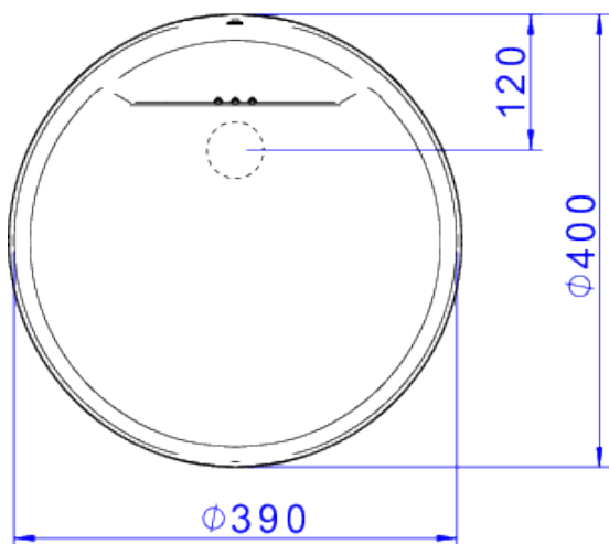
Desenho Técnico
