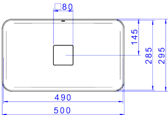
Desenho Técnico
