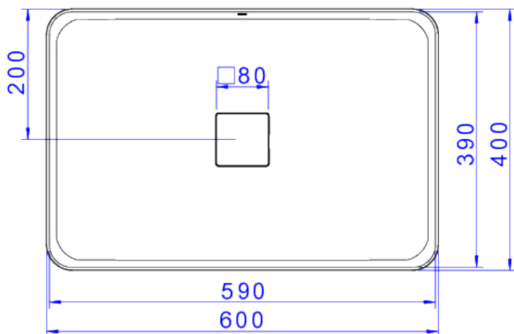
Desenho Técnico
