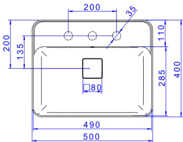
Desenho Técnico
