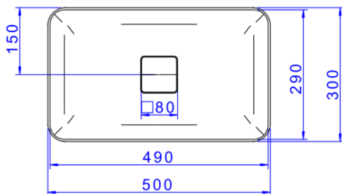
Desenho Técnico
