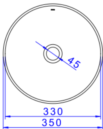
Desenho Técnico
