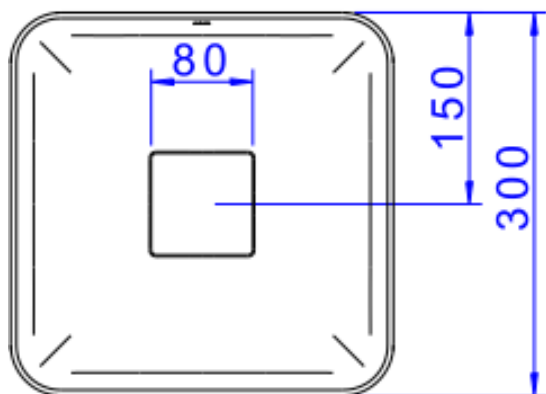
Desenho Técnico
