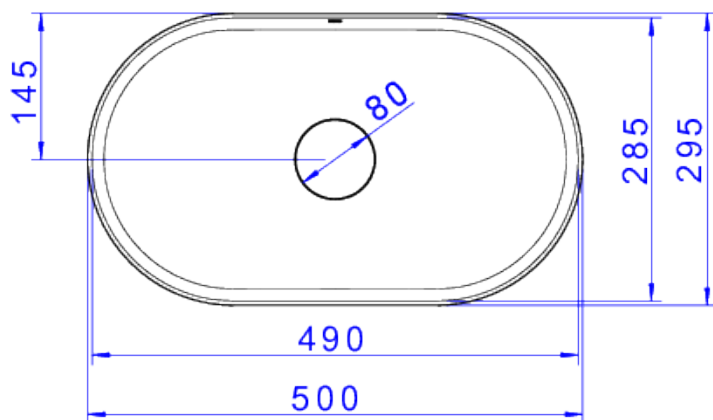
Desenho Técnico
